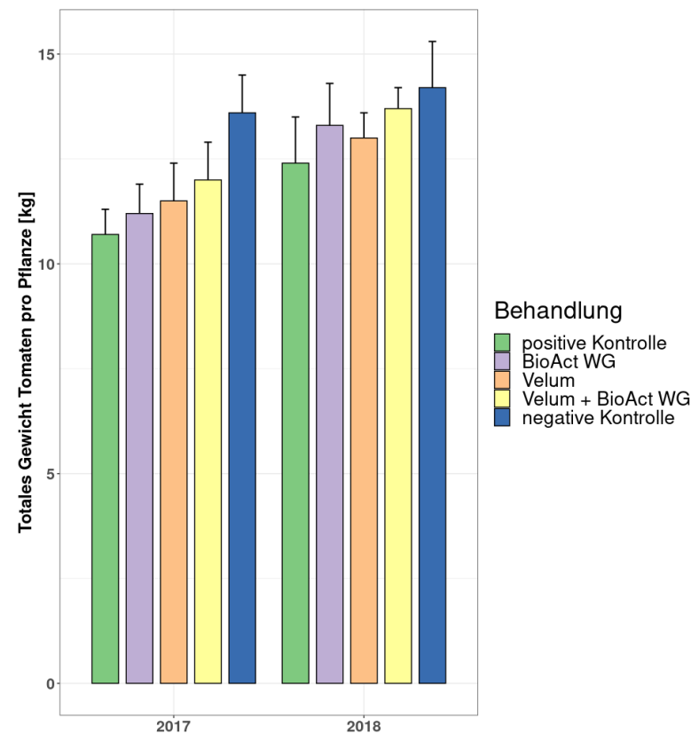
Abbildung 5: Einfluss der Meloidogyne incognita Behandlung mit BioAct WG, Velum und Velum + BioAct WG auf das totale Tomatenerntegewicht pro Pflanze während dem Gewächshausversuch in den Jahren 2017 und 2018. Über 14 Wochen wurde wöchentlich rote Tomaten geerntet und deren Gewicht (kg) und Anzahl bestimmt.
