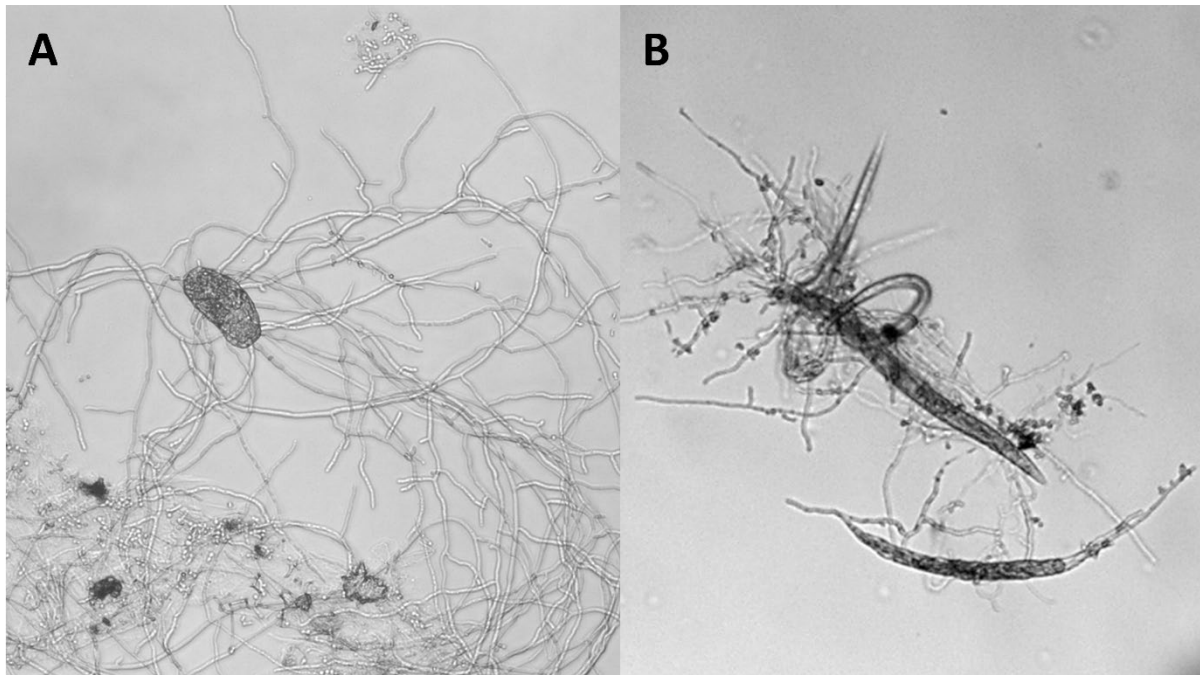
Abbildung 1: Die Pilzfäden und Sporen des Bodenpilzes Pureocillium lilacinum befallen Meloidogyne incognita Eier (A) oder Juvenile des zweiten Larvenstadiums (B).
