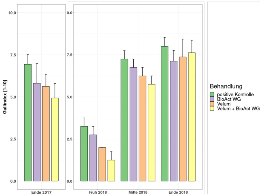
Abbildung 3: Einfluss der Antagonistischen Wirkung von BioAct WG und des chemischen Nematizid Velum gegen Meloidogyne incognita an Tomaten unter Gewächshausbedingungen für die Jahre 2017 und 2018. Der Gallindex der Tomatenwurzeln wurde anhand der Skala von 0-10 nach Zeck (1971) bewertet.
