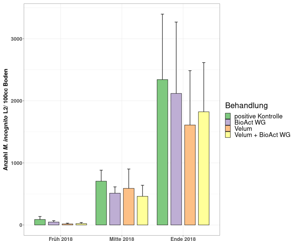
Abbildung 4: Populationsentwicklung von Meloidogyne incognita im Boden in Abhängigkeit von der Behandlung mit BioAct WG, Velum und Velum + BioAct über drei verschiedene Vegetationsphasen (Früh, Mitte oder Ende) im Jahr 2018.
