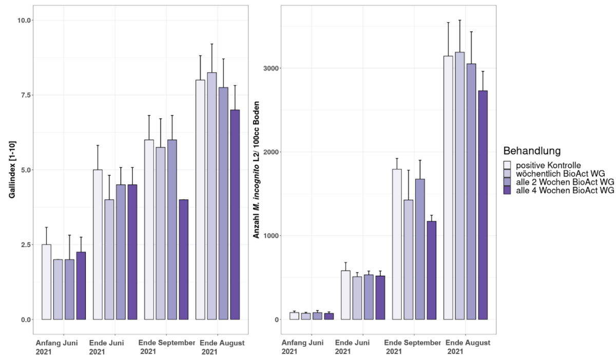
Abbildung 6: Einfluss drei verschiedener Applikationsgaben des biologischen Nematizid BioAct WG gegen Meloidogyne incognita an Tomaten. Entwicklung des Gallindex an Tomatenwurzeln (links) und auf die M. incognita Bodenpopulation (rechts) unter vier verschiedenen Zeitpunkten in der Vegetationsphase 2021. Der Gallindex der Tomatenwurzeln wurde anhand der Skala 0-10 von Zeck (1971) bewertet.
